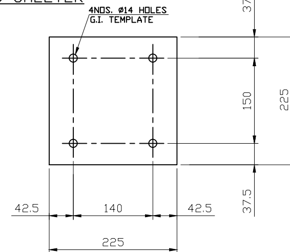
TEMPLATE 225x225x2.5 mm
