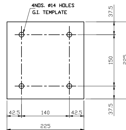
TEMPLATE 225x225x2.5 mm
